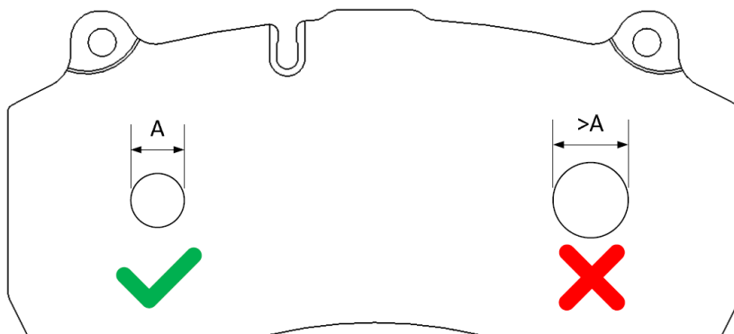
Fig. 1: En la imagen de arriba se muestra una pastilla del freno de disco ModulT. El agujero con la dimensión estándar está representado a la izquierda, y el agujero agrandado se muestra a la derecha.
